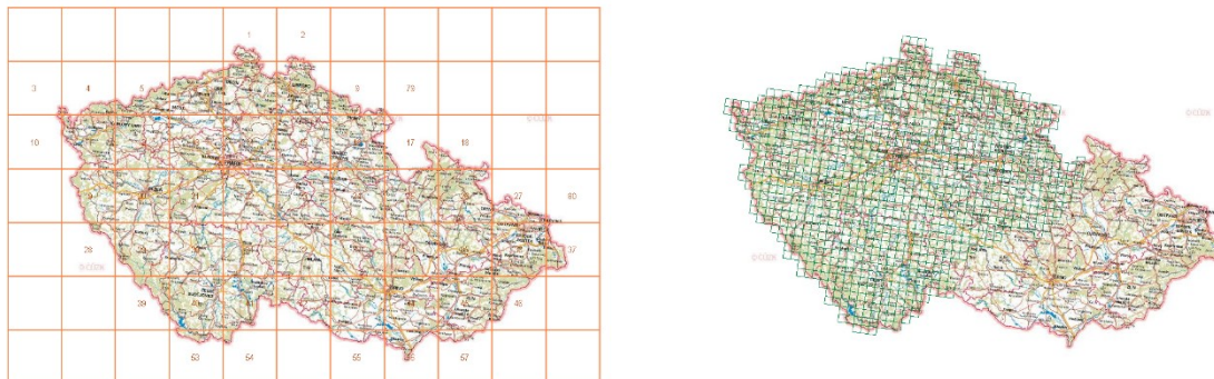
Obr. 18: Klad mapových listů v souřadnicovém systému JTSK v měřítku 1:100000 a klad v souřadnicovém systému Gusterberg v měřítku 1:14400
